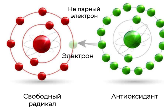
Действие антиоксидантов на свободные радикалы
